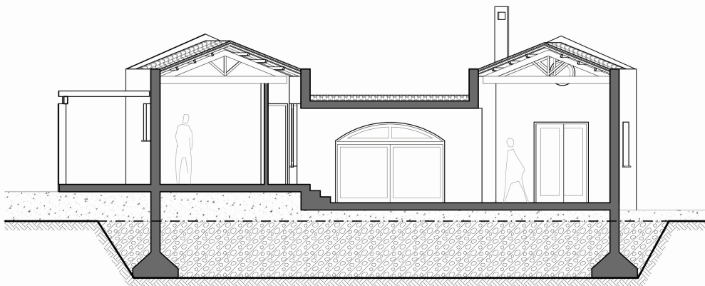
Εικόνα 4: Τομή κατοικίας
